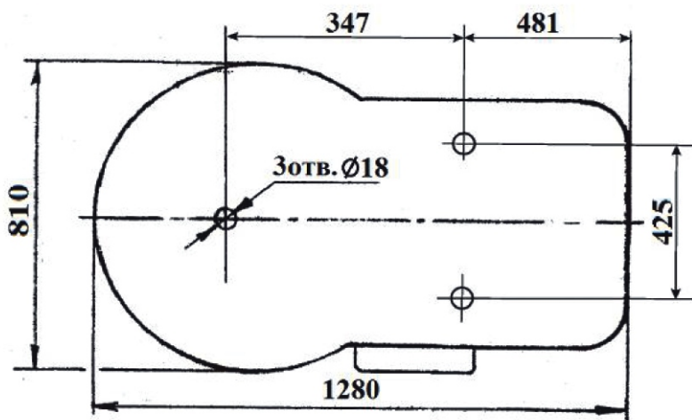
Рисунок 2 - План расположения фундаментных болтов
