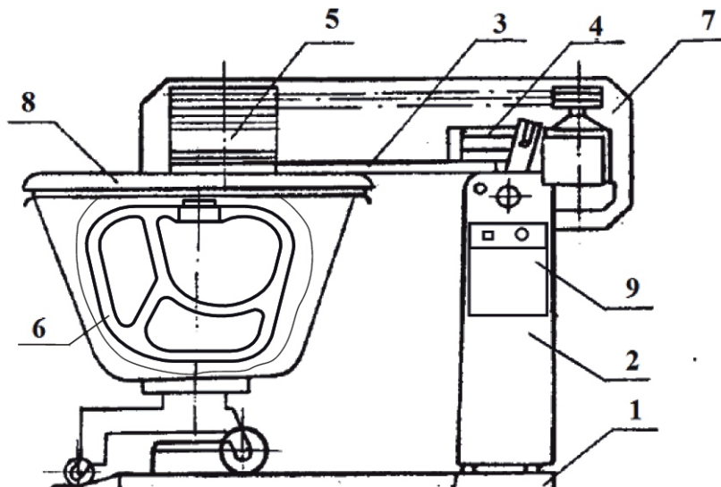
Рисунок 1 - Общий вид тестомеса
