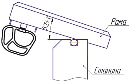
Рисунок 7 - Верхнее положение рамы
