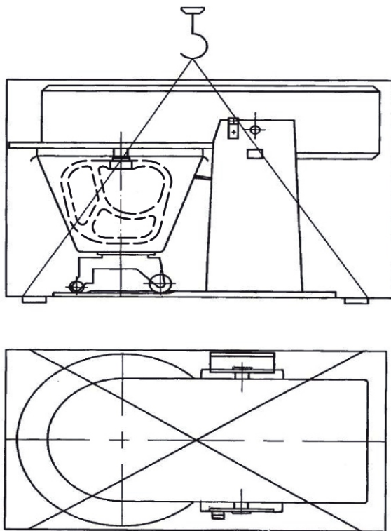
Рисунок 6 - Строровка тестомеса в упаковке
