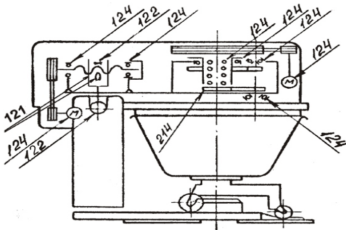
Рисунок 4 - Карта смазки
